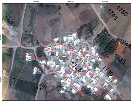
شکل شماره (۷): همپوشانی کروکی موجود با تصویر ماهواره ای و خطوط منحنی میزان
