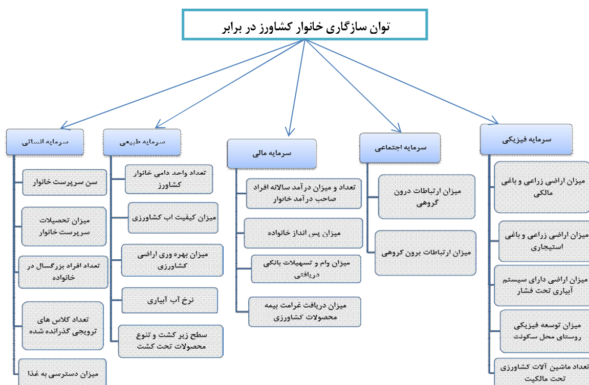
شکل شماره (۱): شاخص توان سازگاری خانوار کشاورز در برابر خشکسالی
