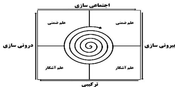
شکل ۱. مدل SECI
