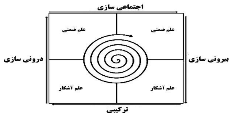
شکل ۱. مدل SECI
