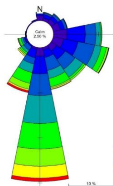
شکل ۵- گلباد هفته اول تا چهارم نمونه برداری (بالا سمت چپ)، گلباد ماه پنجم، هفته پنجم تا هفتم نمونه برداری (بالا سمت راست)، گلباد دو ماه ژوئیه و آگوست. Figure 5. Windrose of the first to fourth week of sampling (left), Windrose of the fifth month, fifth to seventh week of sampling (middle) and Windrose in July and August (right).
