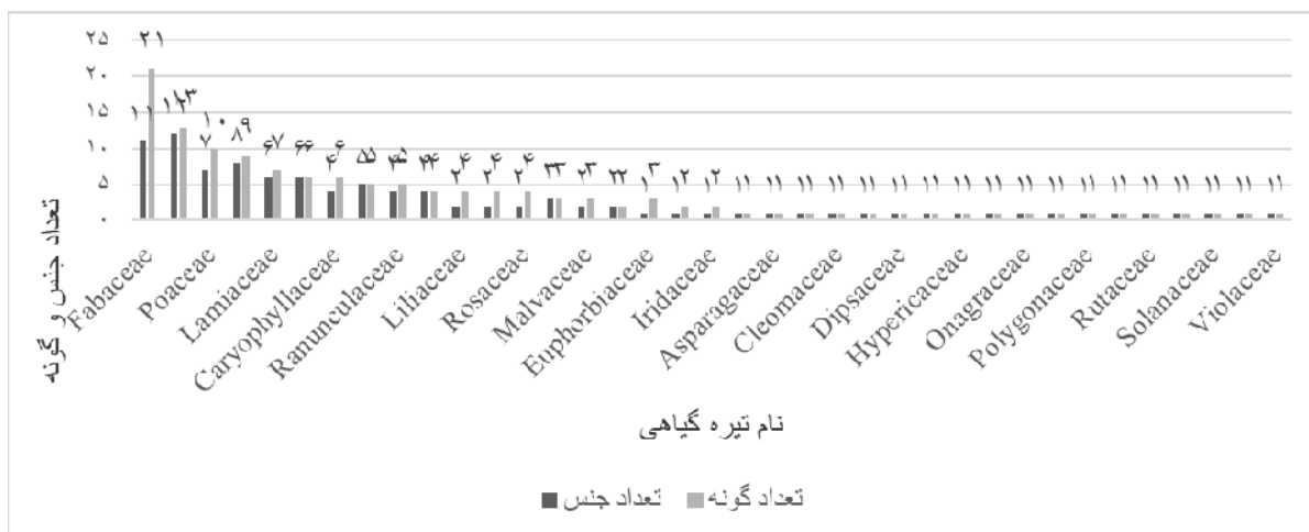
شکل ۸- نمودار تعداد سرده و گونه هر تیره.
