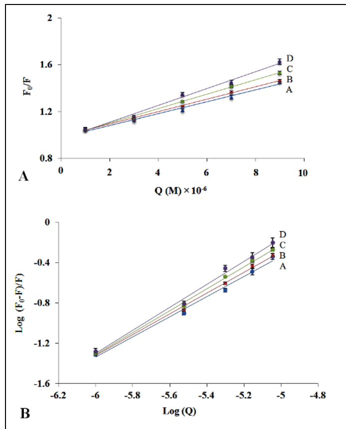
شکل ۴- نمودارهای (A) استرن-وولمر، (B) و هیل در دماهای ۲۹۸ (A)، ۳۰۵ (B)، ۳۱۰ (C) و ۳۱۵ (D) کلوین.
