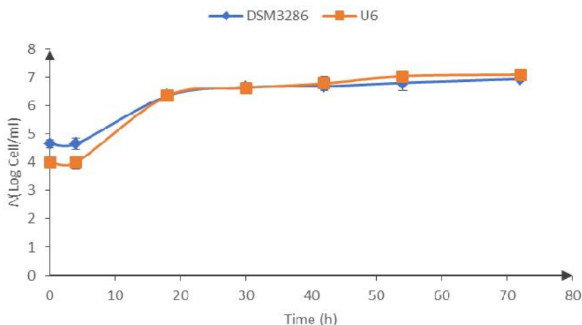
شکل ۵- منحنی رشد سلول‌های طبیعی DSM3286 و جهش یافته U6 مخمر Yarrowia lipolytica در محیط تبدیل زیستی. (لوزی آبی) سویه طبیعی Yarrowia lipolytica DSM3286. (مربع نارنجی) سویه جهش یافته U6 Yarrowia lipolytica .
