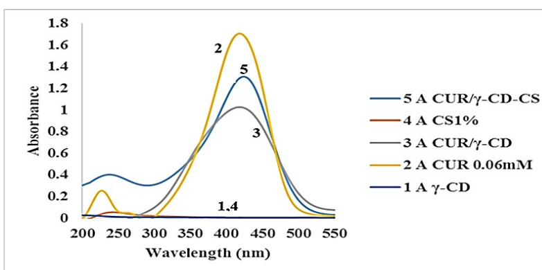
شکل ۲- طیف‌های جذب UV-vis برای \gamma -CD خالص، CUR آزاد در ۴۱۸ nm، کمپلکس CUR/ \gamma -CD، CS ۱ درصد خالص و کمپلکس اصلاح شده CUR/ \gamma -CD-CS در ۴۲۳ nm.
