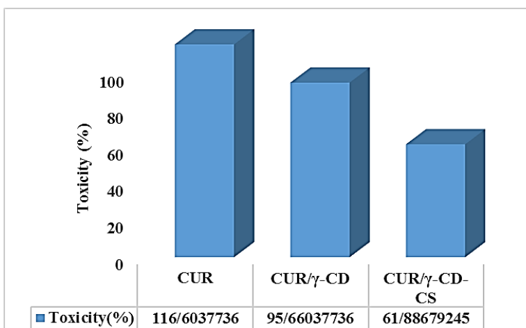
شکل ۱۰- بررسی خاصیت ضدسرطانی CUR، CUR/γ-CD و CUR/γ-CD-CS به روی سلول‌های A549 توسط آزمایش MTT.
