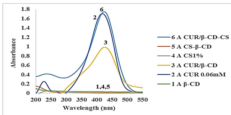
شکل ۱- طیف‌های جذب UV-vis برای \beta -CD خالص، CUR آزاد در ۴۱۸ nm، کمپلکس CUR/ \beta -CD، CS ۱٪ خالص و کمپلکس اصلاح شده CUR/ \beta -CD-CS در ۴۲۴ nm.
