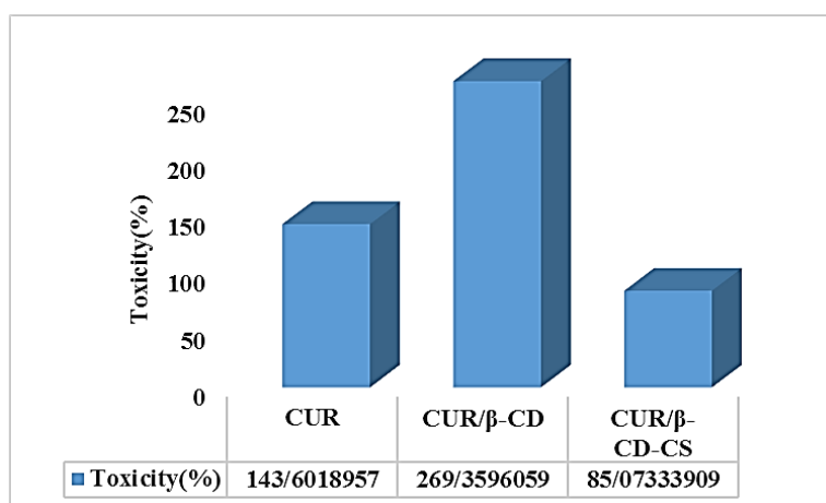
شکل ۹- بررسی خاصیت ضدسرطانی CUR، CUR/β-CD و CUR/β-CD-CS به روی سلول‌های A549 توسط آزمایش MTT.
