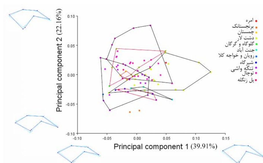
شکل ۸- نمودار تحلیل مؤلفه‌های اصلی ریخت‌سنجی هندسی تارسانگولوم چنگال‌های سمی.
