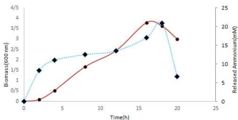
شکل ۲- منحنی رشد و تجزیه اوره توسط جدایه ۶ در محیط TSB حاوی ۵ درصد نمک (■: بیومس، ▲: آزاد سازی آمونیوم و تجزیه اوره).
