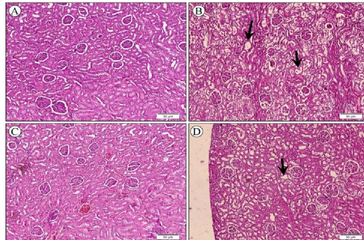
شکل ۱- فوتومیکروگراف برش‌های کلیه A: برش‌های بافتی گروه کنترل ساختار طبیعی را نشان می‌دهند. B: برش‌های بافتی گروه جنتامایسین تخریب بافتی و ریزش اپی‌تلیالی وسیعی را نشان می‌دهد. C: برش‌های کلیه رت‌های تیمار شده با عصاره باباآدم ساختار بافتی نرمال را نشان می‌دهد. D: با تیمار همزمان باباآدم و جنتامایسین، برش‌های کلیه تخریب ملایمی را نشان می‌دهد.
