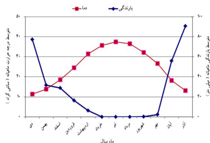
شکل ۳- منحنی آمبروترمیک ایستگاه سینوپتیک بهبهان.
