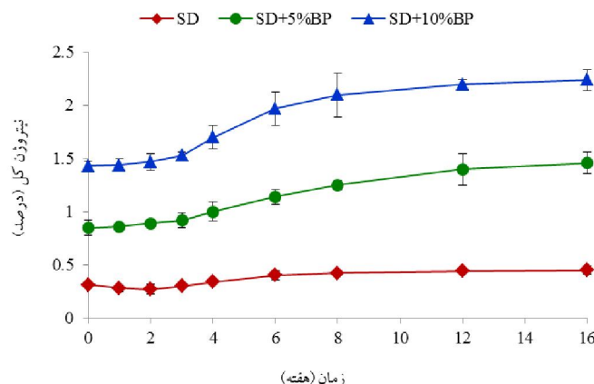
شکل ۵- روند زمانی تغییرات نیتروژن کل خاک‌آاره (SD) تیمار شده با سطوح مختلف پودر خون (BP) طی فرایند ورمی کمپوست سازی.
