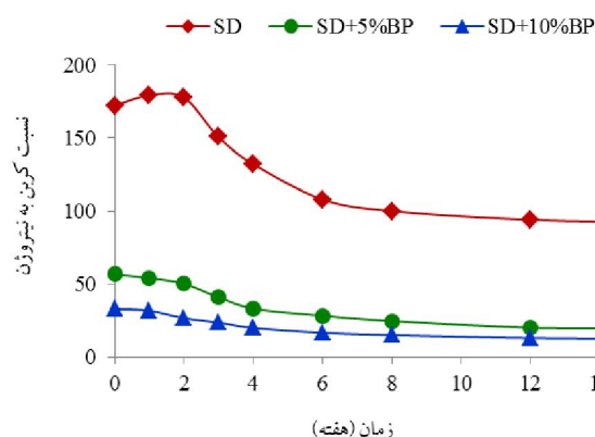
شکل ۶- روند زمانی تغییرات نسبت کربن نیتروژن خاک‌آاره (SD) تیمار شده با سطوح مختلف پودر خون (BP) طی فرایند ورمی کمپوست سازی.
