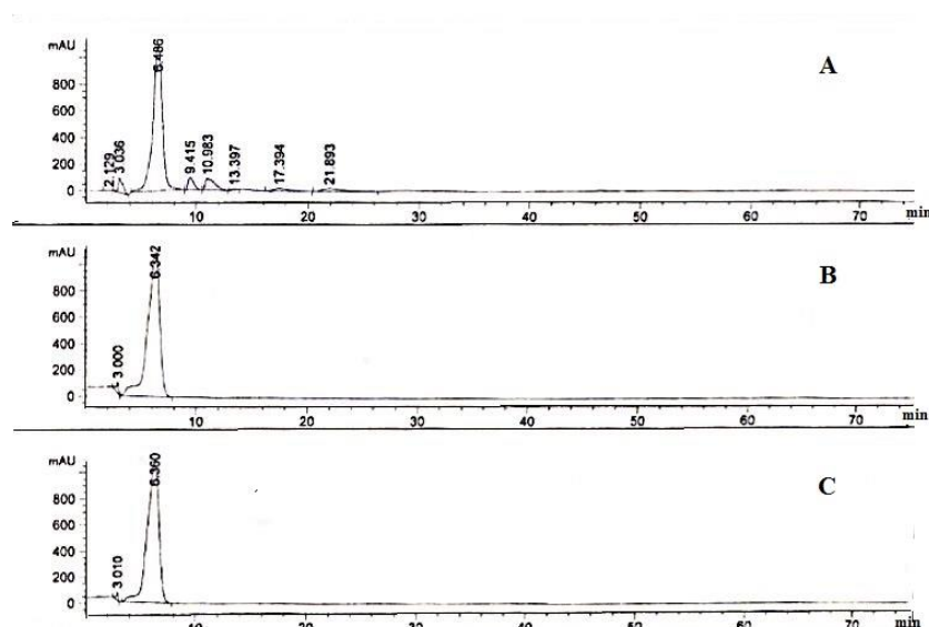
شکل ۴- دیاگرام آنالیز پیکمان بتا کاروتن در دو باکتری S. epidermidis و D. natronolimnaea در مقایسه با بتاکاروتن استاندارد با HPLC. A. S. epidermidis . B. D. natronolimnaea . C. standard beta-carotene.
