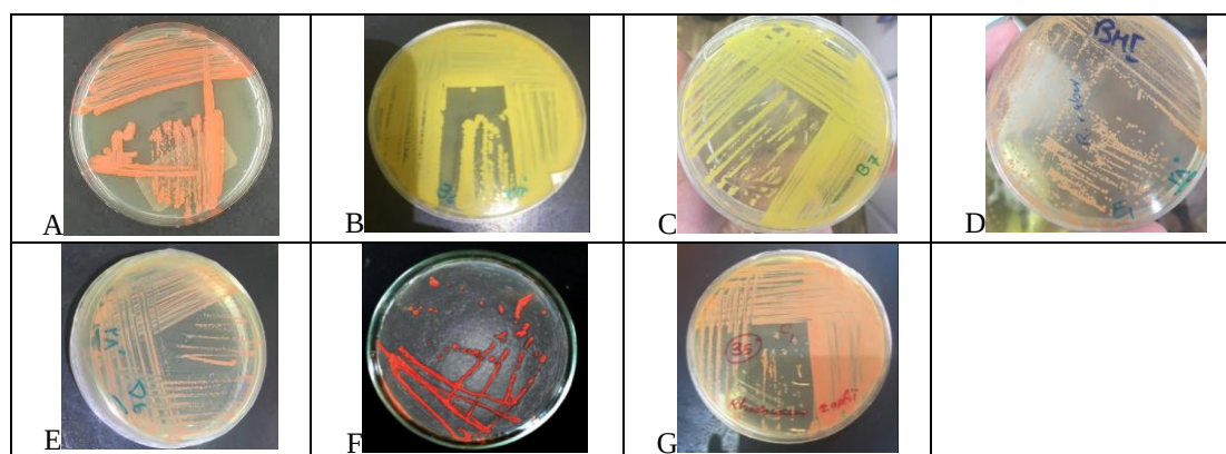
شکل ۲- کلنی‌های باکتری‌های تولیدکننده رنگدانه روی محیط Brain heart infusion (BHI). A. استافیلوکوکوس اپیدرمایدیس. B. میکروکوکوس آلونورا. C. سیتریکوکوس آلكالیتولرانس. D. رودوکوکوس روبور. E. دیتزیا ناترونولیمنا. F. آرتروباکتر اجیلیس، G. رودوکوکوس زوفتی.
