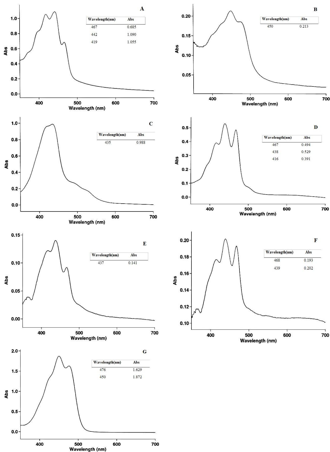
شکل ۳- آنالیز طیف سنجی UV-VIS. A. S. epidermidis . B. A. agilis . C. R. zopfii . D. R. ruber . E. M. aloeverae . F. C. alkaliolerans . G. D. natronolimnaea .
