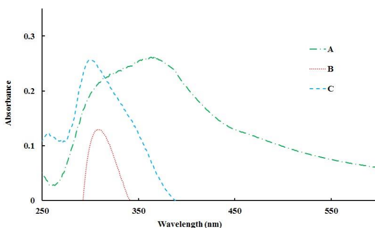
شکل ۱- طیف جذبی UV-Vis نانوذرات مغناطیسی اکسید آهن تولید شده به روش زیستی. A. طیف جذبی سوپرناتانت حاوی نانوذرات تولید شده (سوپرناتانت + آهن (III) کلرید ۶ آبه). B. محلول آبی نمک آهن (محلول آهن (III) کلرید ۶ آبه). C. محلول نمک آهن در محیط کشت NB (محیط کشت NB+آهن (III) کلرید ۶ آبه).
