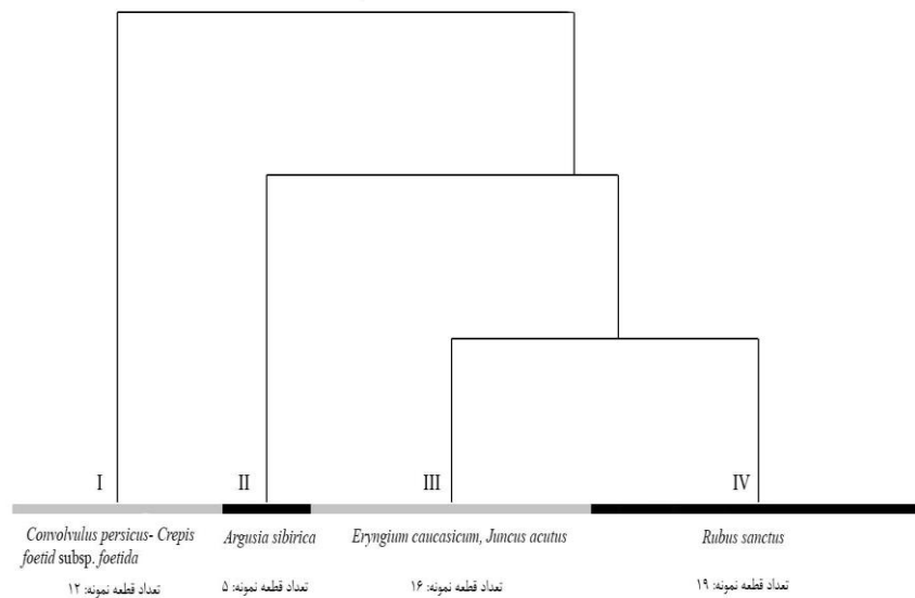
شکل ۳- دندروگرام طبقه بندی قطعات نمونه از طریق Modified TWINSpan. Fig. 3. Cluster analysis of plots by means of Modified TWINSpan
