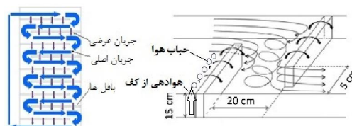
شکل ۲- جریان‌های عرضی و اختلاط بهتر ناشی از نصب مورب بافل‌ها و سیستم هواده‌ای از کف.
