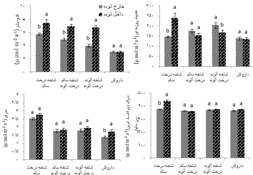
شکل ۳- مقایسه فتوسنتز، هدایت روزنه‌ای، تعرق و میزان دی‌اکسیدکربن بین سلولی در شاخه درخت سالم، شاخه درخت آلوده، شاخه آلوده درخت آلوده و دارویش بین دو موقعیت توده.
