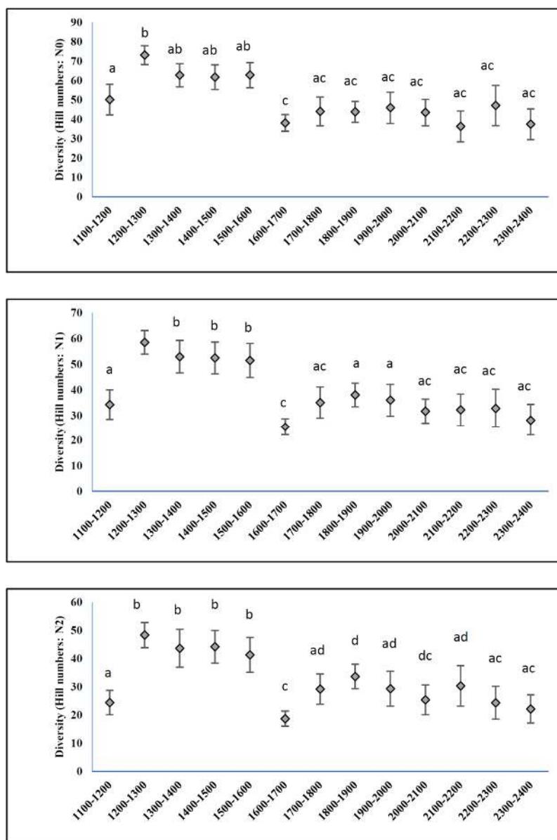
شکل ۹- معنی‌داری آماری شاخص‌های تنوع در طبقات ارتفاعی ۱۰۰ متر در زیر اشکوب اجتماعات گیاهی غرب آلاداغ بر اساس اعداد هیل ( N_0 و N_1 و N_2 ). نوارهای خطا نشانگر محدوده اطمینان ۹۵ درصد است. حروف مشابه در هر نمودار نشانگر عدم وجود اختلاف معنی دار در آن شاخص خاص است.
