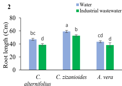
شکل ۲- تأثیر پساب صنعتی بر طول ریشه گیاهان نخل مرداب، وتیور و آلوئه‌ورا.
