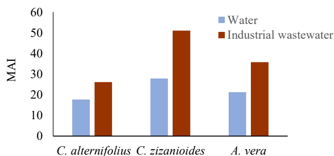
شکل ۱- شاخص انباشت فلزات (روی، کروم، سرب، مس، منگنز، نیکل، منیزیم) در گیاه نخل مرداب، وتیور، آلوئه‌ورا تحت تیمار آب شهری و پساب صنعتی.
