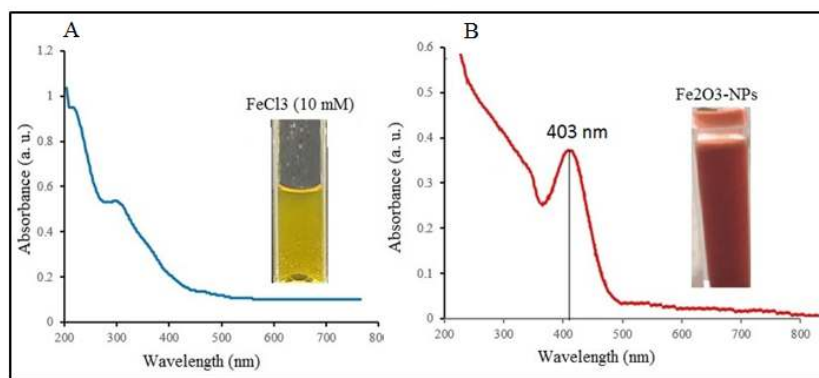
شکل ۱- مشاهدات چشمی و تجزیه و تحلیل‌های اسپکتروفتومتری محلول FeCl 3 در غلظت ۱۰ میلی مولار تحت شرایط دمایی ۲۵ درجه سانتیگراد و دور شیکر ۱۵۰ rpm پس از ۴۸ ساعت انکوباسیون در محیط کنترل (A: تیمار نشده با عصاره عاری از سلول) و واکنش زیست تبدیلی (B: تیمار شده عصاره عاری از سلول).
