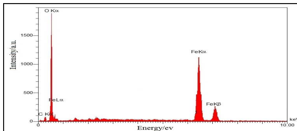
شکل ۸- طیف EDX نانوذرات برون سلولی \text{Fe}_2\text{O}_3 تولیدی بوسیله عصاره عاری از سلول باکتری Alcaligenes sp. strain NV06. Figure 8. Energy dispersive X-ray spectroscopy (EDX) of extracellular magnetite nanoparticles synthesized by CFE of Alcaligenes sp. strain NV06.
