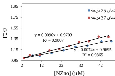
شکل ۶- نمودار ( K_{sv} ) دردمای ۲۵ و ۳۷ درجه سانتی‌گراد.
