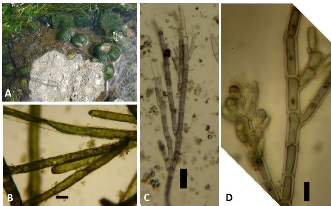
شکل ۷- A. Vaucheria . B. با بزرگنمایی 100x. C. Audouinella eugenea . D. در زیستگاه خود بر روی بستر سنگی. B. با بزرگنمایی 100x. C. Audouinella eugenea . D. با بزرگنمایی 400x همراه با مونواسپورانها. مقیاسها = ۳۰ میکرومتر.
