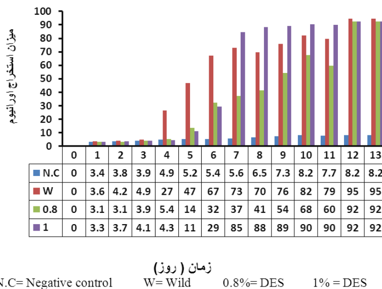
شکل ۱- میزان استخراج اورانیوم توسط باکتری وحشی در مقایسه با باکتری جهش یافته با ۱٪ (V/V) و ۰.۸٪ (V/V) DES (N.C: کنترل منفی، W: باکتری وحشی، ۰.۸٪ (V/V): جهش ناشی از ۱٪ (V/V) DES، ۱٪ (V/V): جهش ناشی از ۰.۸٪ (V/V) DES).
