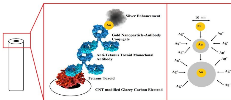
شکل ۱- طرح کلی شناسایی آنتی‌بادی مونوکلونال ضد توکسوئید کزاز با کاربرد تقویت نقره نانوذرات طلا روی الکترود کربن شیشه‌ای اصلاح شده با نانولوله‌های کربنی. Figure 1. The outline for the detection of anti-tetanus toxoid monoclonal antibody by using silver enhancement of gold nanoparticles at carbon nanotubes modified glassy-carbon electrode.
