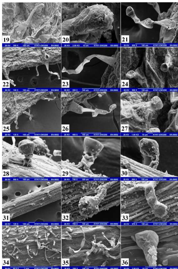
شکل ۲- (۱۹، ۲۰، ۲۱) Gypsophila linearifolia , (۱۹) کرکپوش برگ، (۲۰) سلول رأسی، (۲۱) کرک برگ. (۲۳، ۲۲) Gypsophila melampoda , (۲۲) کرکپوش برگ، (۲۳) کرک برگ. (۲۴، ۲۷) کرک برگ Gypsophila pseudomelampoda . (۲۵، ۲۶) کرک برگ Gypsophila mucronifolia . (۲۸، ۲۹، ۳۰) کرک ساقه Gypsophila pallida . (۳۱، ۳۲، ۳۳) Gypsophila transcaucasica , (۳۱) ساقه کرکپوش، (۳۲، ۳۳) کرک ساقه. (۳۴، ۳۵، ۳۶) Gypsophila perfoliata , (۳۴) کرکپوش ساقه، (۳۵) ساقه کرکپوش، (۳۶) سلول قاعده‌ای.
