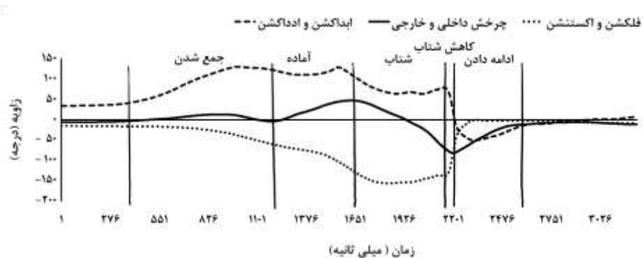
نمودار ۱. تقسیم بندی حرکت سرویس به پنج فاز (جمع شدن، شتاب، کاهش شتاب و ادامه دادن حرکت) طبق زوایای حاصل از شتاب سنج
