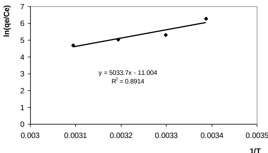
شکل ۵. منحنی تغییرات \ln \left( \frac{q_e}{C_e} \right) بر حسب 1/T برای به‌دست آوردن پارامترهای ترمودینامیکی (غلظت اولیه جذب‌شونده: 0.1 \text{ M} ، دما: 295-323 \text{ K} ، مقدار جاذب: 3/5 \text{ g} ) جدول ۲. پارامترهای ترمودینامیکی جذب فرمیک اسید روی کربن رنگبر
