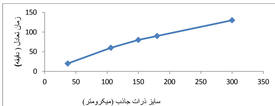
شکل ۳. تأثیر اندازه ذرات جاذب کربن فعال بر زمان تعادل جذب یون نیکل (دمای محیط، دور شیکر ۱۵۰ rpm، غلظت ۰/۱۰ ppm گرم کربن فعال، pH=۶)
