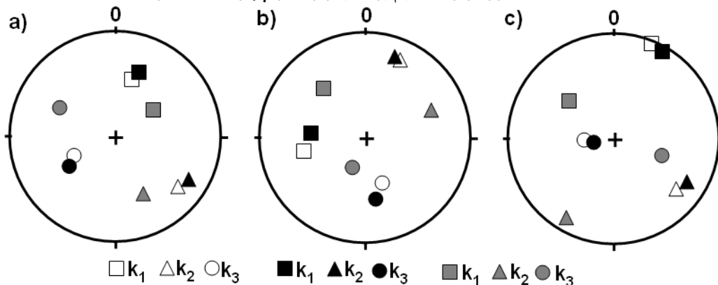
شکل ۵. جهت‌یابی محوره‌های AMS (سفید)، و HFA به جدایش پارامگنتیک (سیاه) و فرومگنتیک (خاکستری) با ترسیم هم‌زمان این محورها می‌توان دریافت که محوره‌های پارامگنتیک نسبت به محوره‌های فرومگنتیک سازگاری بیشتری با محوره‌های AMS دارند. a، b و c به ترتیب نمونه‌های ۲b۳، ۱b۲۷ و ۲b۶۸ هستند. به نظر می‌رسد محوره‌های فرومگنتیک نسبت به AMS چرخیده است.
