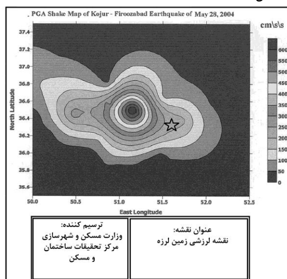
شکل ۱۰. نقشه لرزشی زمین‌لرزه بلده-کجور (برگرفته از گزارش شماره ۲ مرکز تحقیقات ساختمان و مسکن) با توجه به این نکته که b-value مربوط به لرزه‌خیزی پس‌زمینه که پس از حذف خوشه‌های لرزه‌ای به دست می‌آید، می‌تواند محل تنشگاه‌ها را نشان دهد، این خوشه‌ها (پیش‌لرزه و پس‌لرزه) از بین داده‌ها حذف شد. سپس نقشه
