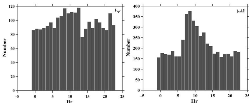
شکل ۳. هیستوگرام تعداد زمین‌لرزه‌ها در ساعات شبانه روز: الف) برای زمین‌لرزه‌های با M \geq 1.7 و ب) M \geq 2.1
