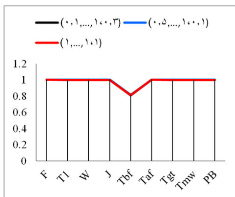
شکل ۶. اندازه و توان آزمون برای ۶ تیمار و اندازه نمونه (۴، ۸، ۱۲، ۲۴، ۳۰، ۴۰)
