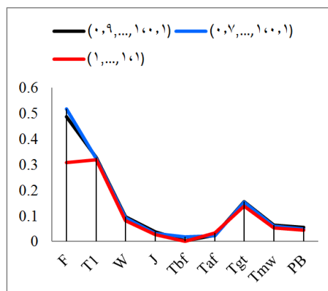
شکل ۷. اندازه و توان آزمون برای ۱۰ تیمار و اندازه نمونه (۵، ۵، ۵، ۵، ۵، ۵، ۵، ۵، ۵، ۵)
