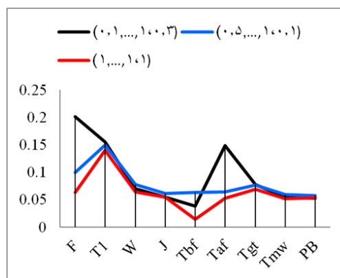
شکل ۶. اندازه و توان آزمون برای ۶ تیمار و اندازه نمونه (۴، ۸، ۱۲، ۲۴، ۳۰، ۴۰)
