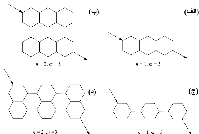
شکل ۱. چند مورد از نانونوارهای گرافن که از یک جایگاه در سمت چپ و از جایگاه متقابل در سمت راست به دو زنجیره اتمی متصل شده‌اند. الف) و ب) موارد زیگزاگ و ج) و د) موارد دسته صندلی را نشان می‌دهند. n و m به ترتیب نشان‌دهنده طول و عرض نانونوار هستند
