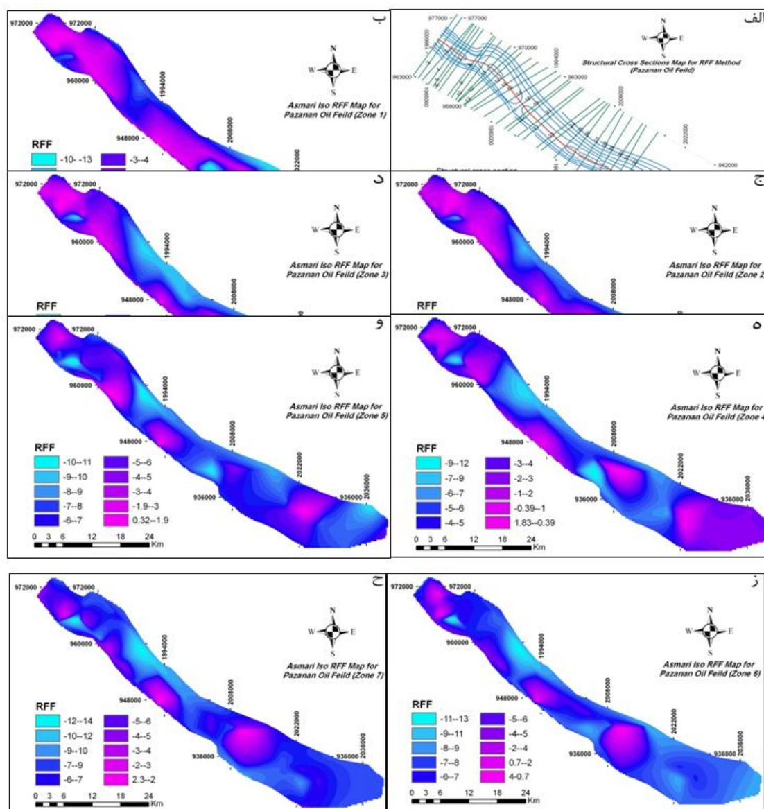
شکل ۶. الف) موقعیت برش‌های عرضی تهیه شده بر روی سرسازند آسماری میدان نفتی پازنان برای به‌کارگیری روش RFF. ب تا ح) به‌ترتیب نقشه‌های هم‌م RFF برای سرسازند آسماری، عمق منطبق بر میانه پهنه‌های یک، دو، سه و چهار و پنج و شش و هفت سازند آسماری (مناطق قرمز رنگ نواحی دارای حداکثر تراکم شکستگی را نشان می‌دهند)
