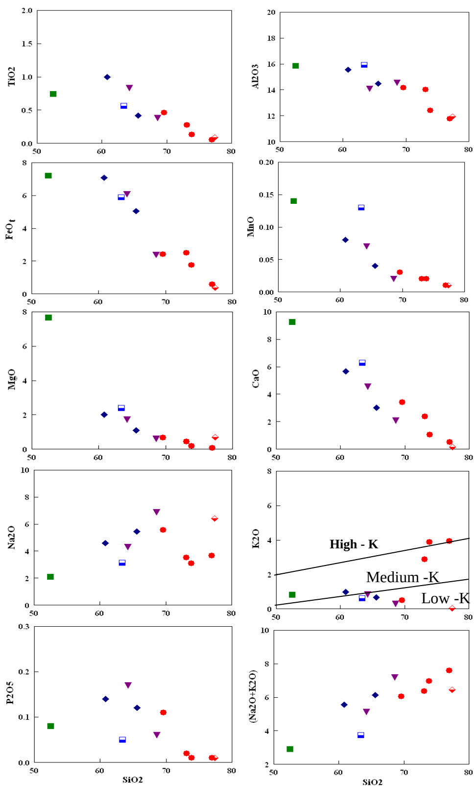
شکل ۷. نمودارهای تغییرات اکسید عناصر اصلی در برابر \text{SiO}_2 ، نمادها نظیر شکل ۴ هستند
