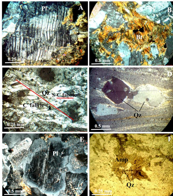
شکل ۲. A) خمیدگی ماکل‌ها در پلاژیوکلاز (Pl) مربوط به یک نمونه کوارتز دیوریتی در نور XPL، B) بلور بیوتیت (Bt) که شدیداً چین‌خورده (مجدد) است (در نور XPL). با وجود دگرشکلی شدیدی که در این‌جا اعمال شده پلاژیوکلازها (Pl) همچنان به‌صورت تیغه‌های کشیده در مقطع حضور دارند، C) بلورهای شدیداً دگرشکل یافته از کوارتز (Qz) همراه فابریک‌های S-C و C' در این تصویر مشخص شده‌اند (در نور XPL)، D) بافت چشمی در بلورهای کوارتز (Qz) در نمونه مربوط به گرانیتوئید میلونیتی درویشان (در نور XPL)، D) پلاژیوکلاز با منطقه‌بندی نوسانی و حاشیه‌های خورده شده در یکی از نمونه‌های آنکلاو (در نور XPL) و F) تشکیل آمفیبول (Amp) در اطراف بلورهای کوارتز (Qz) (در نور PPL)
