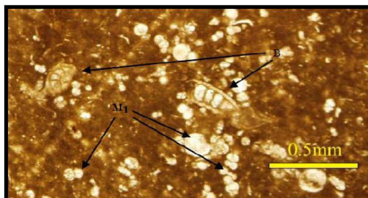
شکل ۱۴. افزایش درصد فرامینفرهای بنتیک (B) و مورفوتایپ نوع اول (M1) نشان دهنده مرز سکاسی از نوع دوم در نمونه G30
