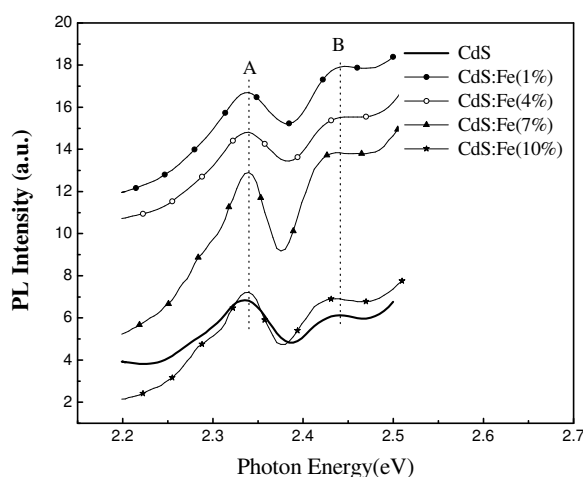
شکل ۵. طیف لومینسانس نانوذرات CdS با نسبت‌های مختلف آلاینش ( [TG] = 0.09 \text{ M} ). انرژی برانگیختگی 3.45 \text{ eV} است.
