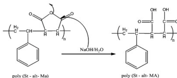
شکل ۱. مکانیسم تبدیل کوپلیمر (استایرن-متناوب-مالئیک انیدرید) به کوپلیمر (استایرن-متناوب-مالئیک اسید)
