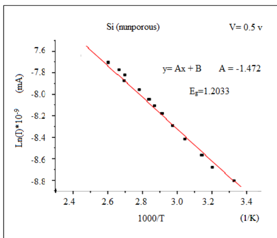
شکل ۶. a) نمودار اندازه‌گیری گاف انرژی نمونه قبل از تخلخل. گاف انرژی محاسبه شده برابر با ۱/۲۰۳۳ است
