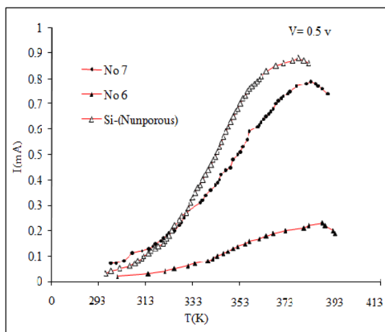
شکل ۵. نمایش تغییرات جریان با دما برای دو نمونه ۶ و ۷ و نمونه متخلخل نشده در ولتاژ V = ۰/۵ مشاهده می‌شود که رسانندگی نمونه پس از تخلخل کاهش پیدا کرده است
