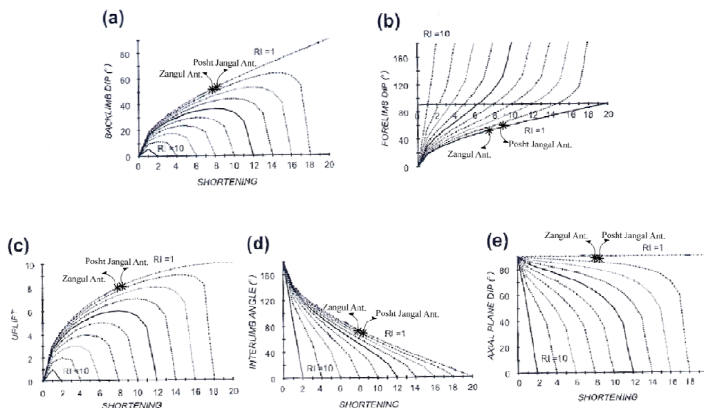
شکل ۱۰. نمودارهای تعیین پارامترهای هندسی چین‌های جدایشی [۸]. منحنی‌های نمودارها، منطبق بر مقادیر RI به ترتیب ۱، ۱.۱۱، ۱.۲۵، ۱.۴۳، ۱.۶۷، ۲، ۲.۵۰، ۳.۳۳ و ۱۰ هستند. (موقعیت تاق‌پس زنگول بر مبنای پارامترهای هندسی آن به صورت ستاره در نمودارها نمایش داده شده است)
