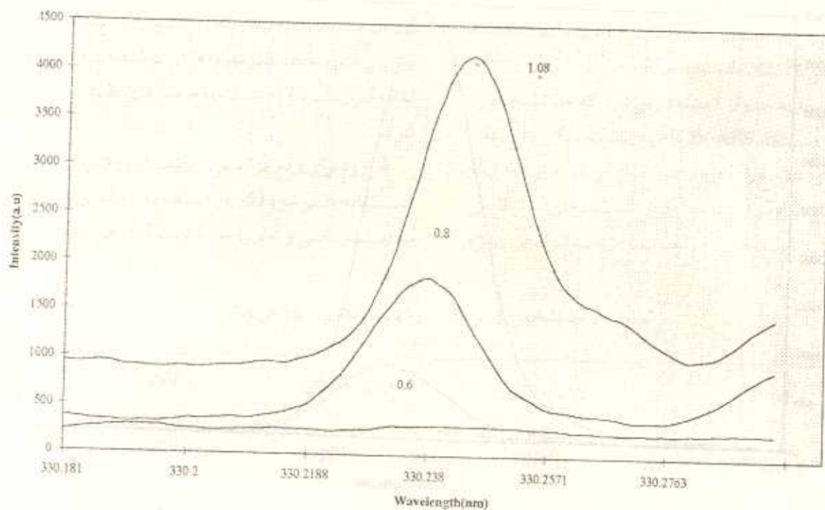
شکل ۳- اثر تغییرات توان پلاسما بر حسب کیلووات بر روی شدت نشر محلول 10 \text{ ppm Zn} + 300 \text{ ppm Na}
