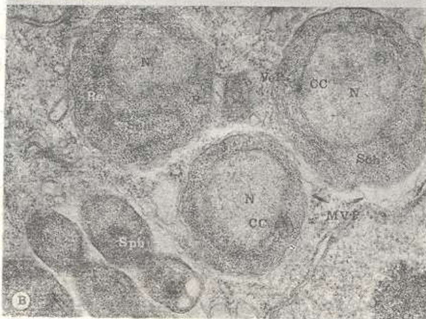
شکل ۳ - باکوله آدافنیه: شیزونت با هسته‌های در شروع تقسیم ، 60000 \times A و 33000 \times B . مرکز ، MP = غشا پلاسمیک ، MVP = غشا واکوئل انگلی ، N = هسته ، R = ریبوزومها ، جنیشی CC = کیسکهای قطبی شده ، VeP = سپروبلست ، Sph = شیزونت ، Sch = شبکه داخل سینوپلاسمی Re
