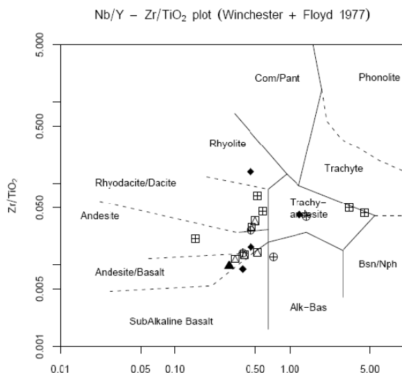
شکل ۶. نمودار Zr/TiO_2 در مقابل Nb/Y [۱۱]، بر مبنای این نمودار سنگهای آتشفشانی منطقه آشتیان در قلمرو بازالت ساب آکالن، آندزیت، آندزیت، تراکی آندزیت، داسیت، ریوداسیت و ریولیت قرار گرفته‌اند
