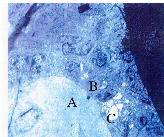
شکل ۵. میکروگراف از تخمدان موش آزمایشی (بزرگنمایی \times 2000 ) -A هسته اووسیت -B سلول فولیکولر -C واکنش
