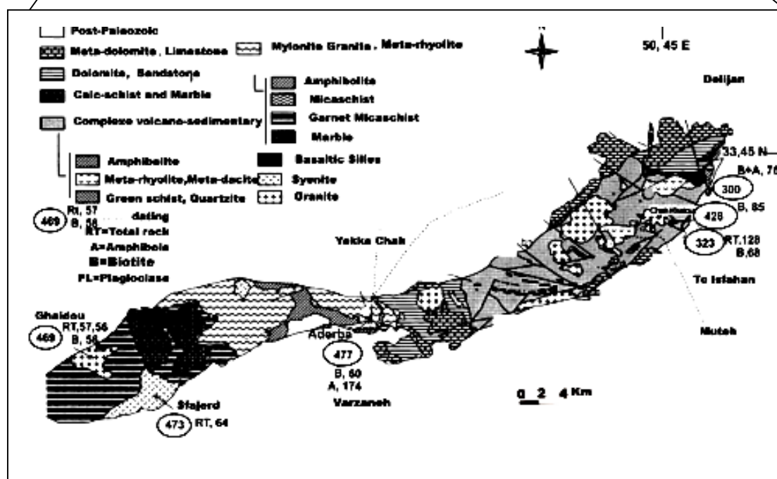
شکل ۲. نقشه زمین‌شناسی منطقه شمال شرق گلیایگان همراه با تعیین سن ایزوتوپی برخی از نمونه‌ها [سن گرانیات قیدو=(۵۷ Ma)، میلونیت گرانیات ورزنه=(۶۰ Ma)، گرانیات چاه خاتون=(۱۲۸ Ma)، متابازالت=(۸۵ Ma) و کمپلکس ولکانوسدیمتر=(۷۶ Ma) میلیون سال قبل]، اقتباس از رشیدنژاد [۸]. همراه با برخی تصحیحات سنگ‌شناسی.
