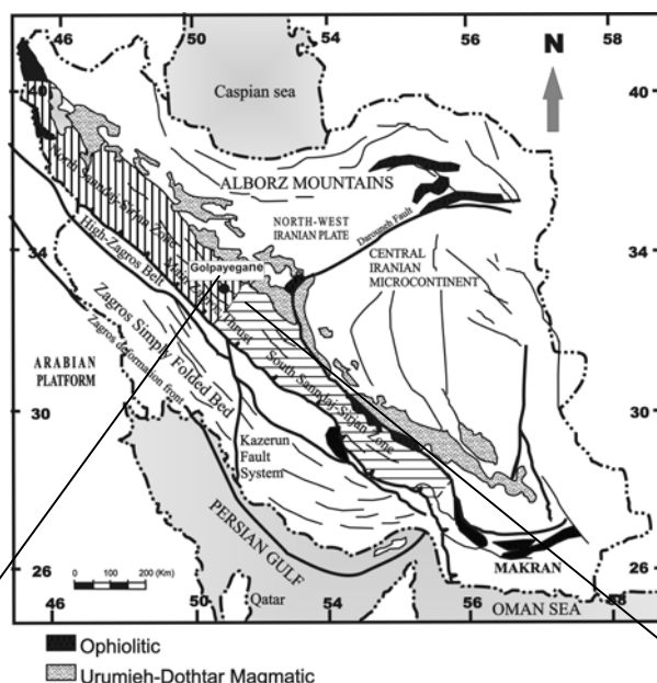
شکل ۱. نقشه واحدهای تکتونیکی ایران همراه با موقعیت منطقه بررسی شده در زون سنج-سیرجان.
