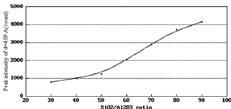
شکل ۱۲. تغییرات شدت پیک ۴.۰۹ Å به ازای نسبت SiO 2 /Al 2 O 3
