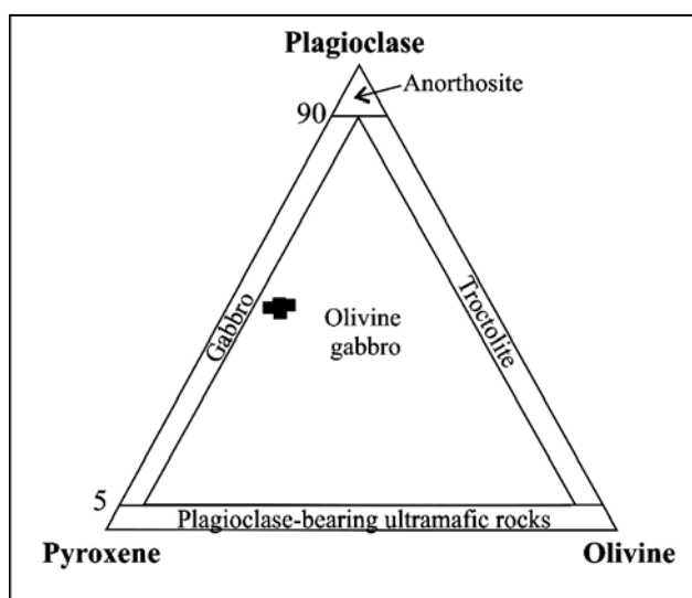
شکل ۵- الف) نمونه‌های بازیک توده نفوذی شکر ناب بر روی نمودار پلاژیوکلاز-کلینوپیکروکسن-اولیوین در محدوده الیوین گابرو [۸] قرار می‌گیرند
