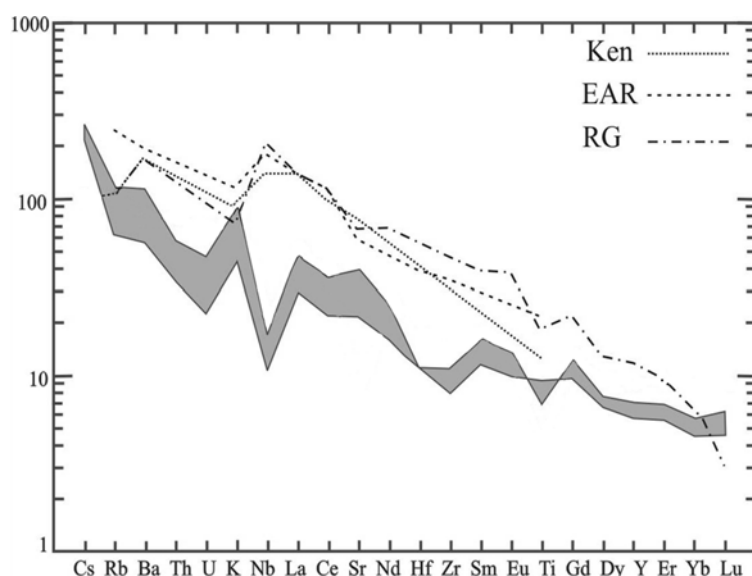
شکل ۱۰- نمودار عنکبوتی نمونه‌های توده نفوذی شکرناپ با نمونه‌های مربوط به برخی از مناطق ریفت دنیا مقایسه شده است. نمونه‌ها همگی نسبت به گوشته اولیه نرمالیزه شده‌اند. محدوده خاکستری مربوط به توده نفوذی شکرناپ، EAR معرف ریفت شرق آفریقا [۲۶]، Ken معرف ریفت کنیا [۲۶] و RG معرف ریفت راین واقع در مرکز آلمان [۲۷] هستند
