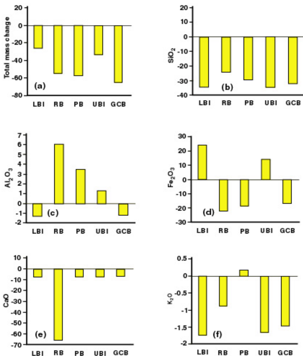
شکل ۵- تغییرات جرم کلی (a) و عناصر Si (b), Al (c), Fe (d), Ca (e), K (f) در واحدهای بوکسیتی قپی
