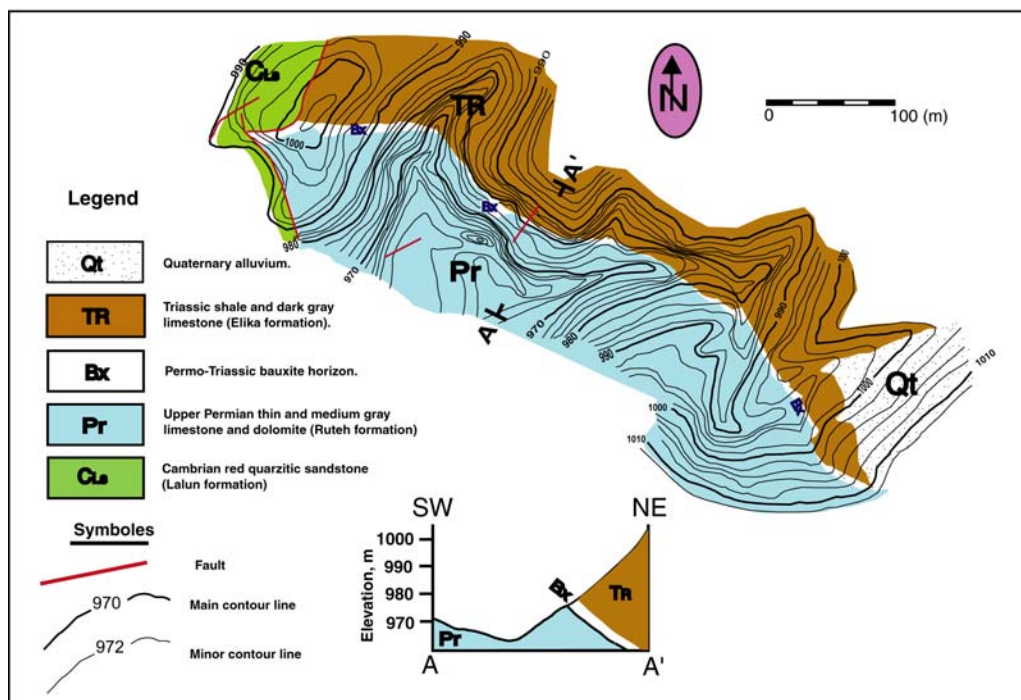
شکل ۱- نقشه زمین شناسی به همراه یک مقطع عرضی از منطقه قبی (به نقل از کلاگری و همکاران، ۱۳۸۲)
