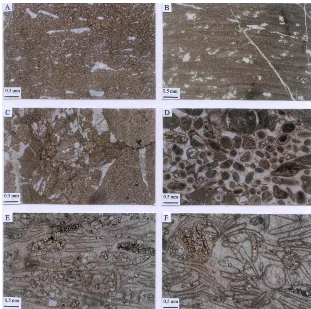
شکل ۴- A- دولومدستون با فابریک چشم پرنده‌ای مربوط به رخساره C، مقطع توسط الیزارین قرمز رنگ‌آمیزی شده است (نمونه برش گذار سرخ) B- دولومدستون لامینه‌دار با فابریک چشم پرنده‌ای و قالب‌های دروغین ژپس و انیدریت در رخساره C، مقطع توسط الیزارین قرمز رنگ‌آمیزی شده است (نمونه از برش اسلام‌آباد) C- گرینستون اینتراکلاستی از رخساره طوفانی کربناته، در این تصویر، اینترکلاست‌های میکریتی بوده‌اند و فابریک سیمان از نوع هم بعد است. بالای مقطع به سمت چپ عکس است بنابراین ساختمان رسوبی از نوع لایه‌بندی تدریجی نیز در اینجا مشاهده می‌گردد (نمونه از برش گذار سرخ) D- گرینستون الیدی اینتراکلاستی مربوط به رخساره طوفانی کربناته. الیدها دارای فابریک‌های شعاعی و متحد‌المرکز هستند. فابریک سیمان نیز غالباً از نوع هم بعد است (نمونه از برش گذار سرخ) E- گرینستون بیوکلاستی الیدی از رخساره طوفانی کربناته. الیدها دارای فابریک متحد‌المرکز بوده و دوکفه‌ای‌ها نیز توسط کلسیت اسپاری پر شده‌اند. فابریک‌های سیمان از نوع دروزی موزائیکی و هم قعد هستند بلورهای اتومورف دولومیت نیز به وضوح دیده می‌شوند. برخی از آنها حالت زونه مانند نیز دارند (نمونه از برش گذار گچال) F- گرینستون بیوکلاستی در رخساره طوفانی کربناته. بیوکلاست‌ها شامل دوکفه‌ای و شکم‌پایا دیواره اسپاریتی هستند. فابریک‌های سیمان از نوع هم بعد و دروزی موزائیکی‌اند جانشینی بلورهای اتومورف دولومیت در برخی از آوکه‌ها دیده می‌شوند (نمونه از برش گذار گچال)
