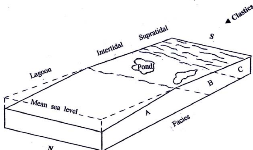
شکل ۸- مدل رسوبی سازند سرخ شیل در منطقه بررسی شده. این مدل بیان‌گر رمپ کریناته- تخریبی است. رخساره‌های سیلیسی آواری در بخش جنوبی حوضه از گسترش زیادی برخوردارند. به سمت مرکز حوضه از ضخامت آن‌ها کاسته شده و در بخش شمالی حوضه، رخساره‌های کریناته فزونی می‌یابند
